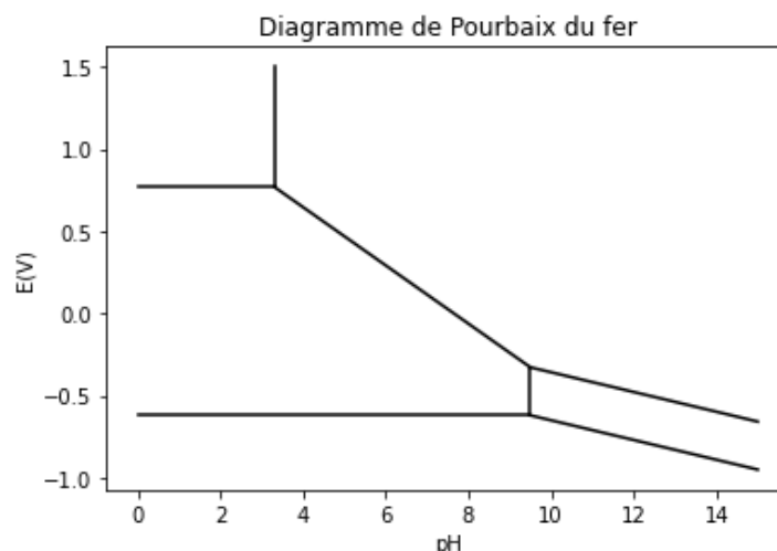
Figure 7 - Diagramme de Pourbaix du fer
