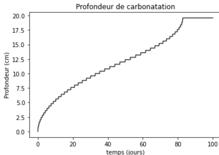
Figure 5 - Évolution de la profondeur du front de carbonatation au cours du temps
