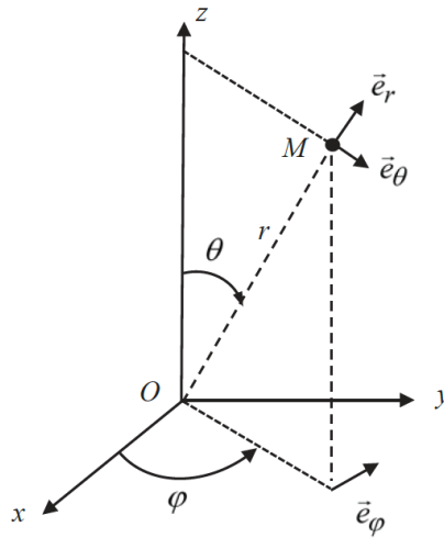
Figure 3 - Coordonnées sphériques
