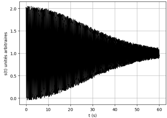
Figure 6b - Interférogramme
