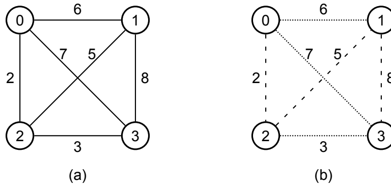
Figure 5 - (a) Le graphe correspondant au réseau de l'île de Korbe. (b) Exemple de configuration finale (contrôlée par MaxDébit) atteinte à l'issue d'une partie. Les arêtes choisies par le joueur MaxDébit sont représentées par un trait discontinu et celle par le joueur MinLatence par une ligne en pointillés
